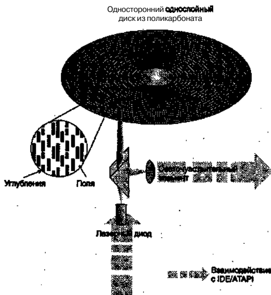
Рис. 3.4. Принцип действия дисковода CD-ROM
