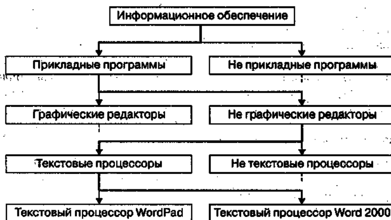
Рис. 1.6. Пример, поясняющий принцип действия метода дихотомии
